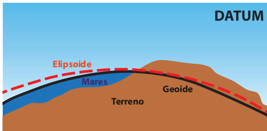
Figura 2.7. Representación esquemática de los componentes de un sistema de referencia (elipsoide, geoide y Datum).
