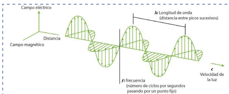
Figura 1.2. Características de la energía electromagnética
