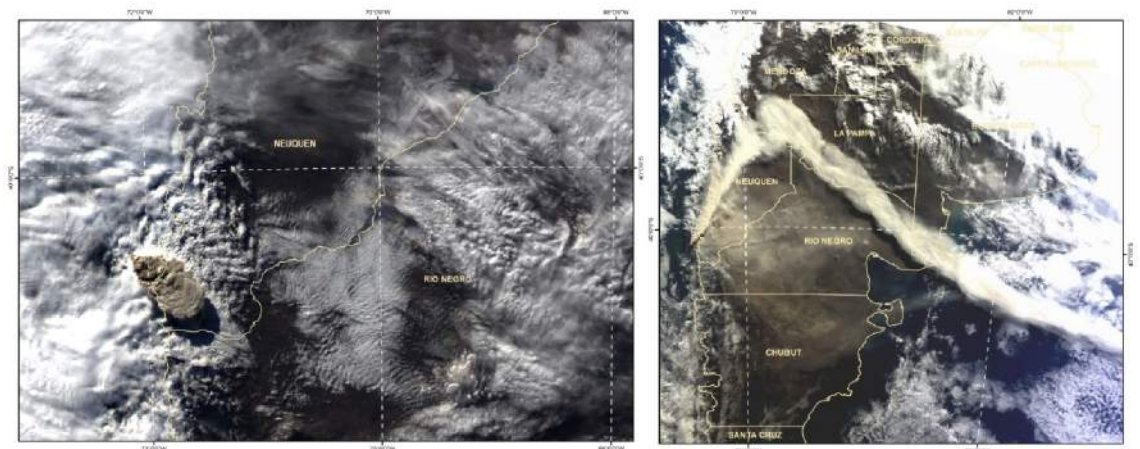
Figura 1.15. Erupción del Complejo Volcánico Puyehue-Cordón Caulle (Chile). Imágenes Sensor MODIS. Izq. Imagen MODIS Aqua, Fecha: 4 de junio de 2011. Der. Imagen MODIS Terra. Fecha: 6 de junio de 2011.
