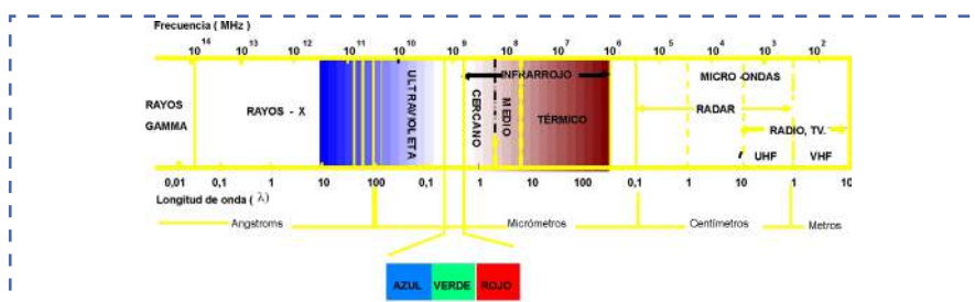
Figura 1.3. Espectro electromagnético ordenado de menor (izq.) a mayor (der.) longitudes de onda (parte inferior) y de mayor (izq.) a menor (der.) frecuencia (parte superior).
